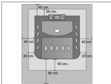
Vista superior, distancias a respetar
